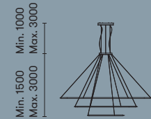
H Ø2000 mm 224W Ø1200 mm 18720 lm Ø600 mm
