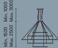
F Ø600 mm 328W Ø1200 mm 27360 lm Ø2000 mm Ø1200 mm Ø600 mm
